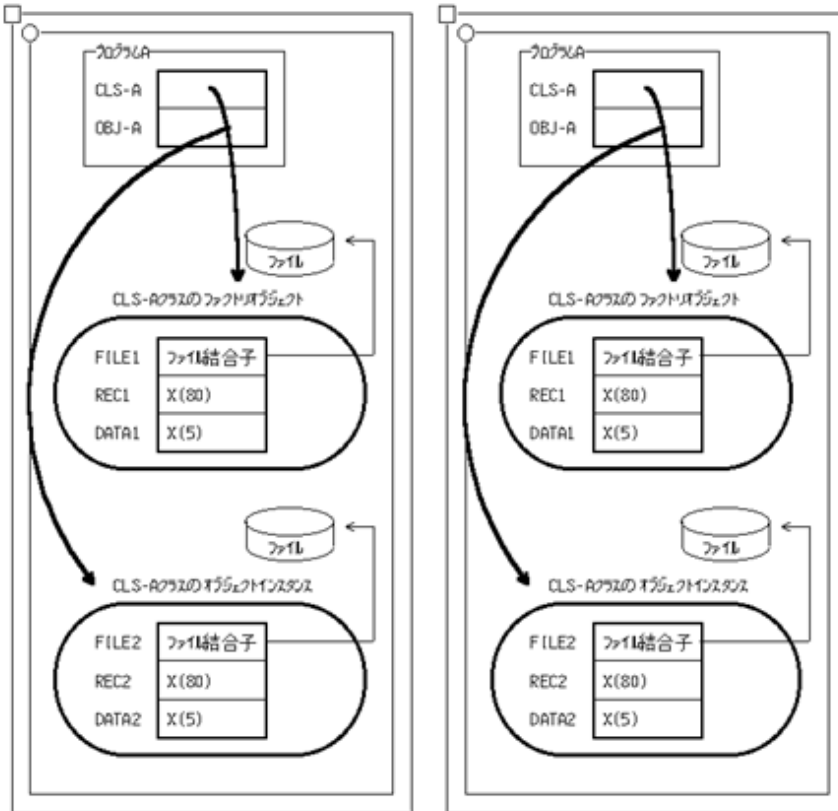
図18.4 シングルスレッドプログラム
