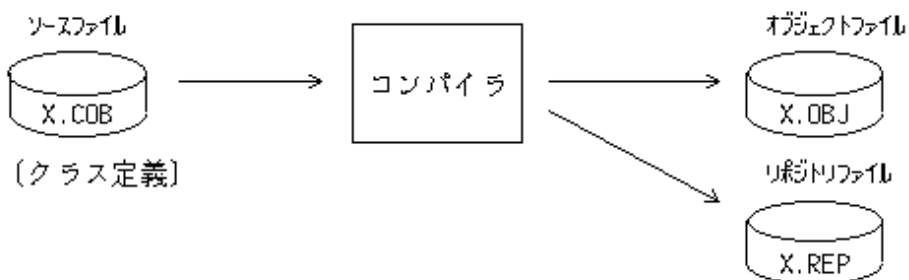
図16.7 リポジットリファイルの出力
