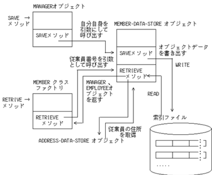
図16.21 保存/復元の処理の流れ
