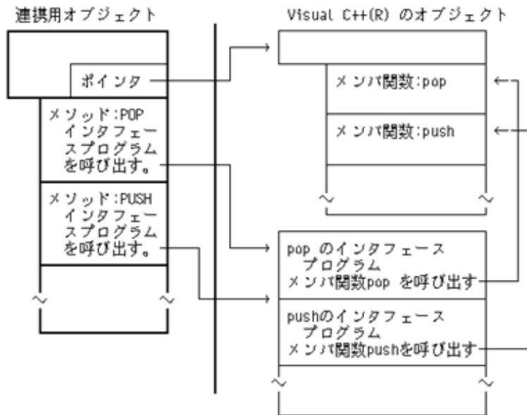
図16.12 インタフェースプログラムの構造
