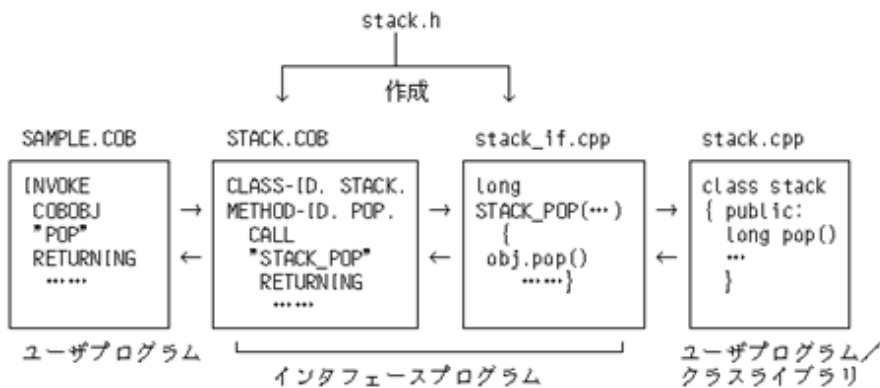
図16.11 インタフェースプログラムのイメージ
