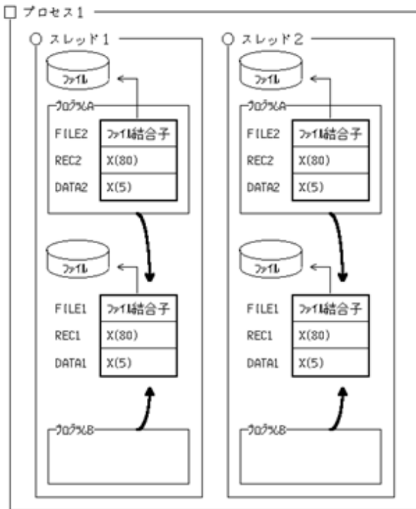
図18.3 マルチスレッドプログラム
