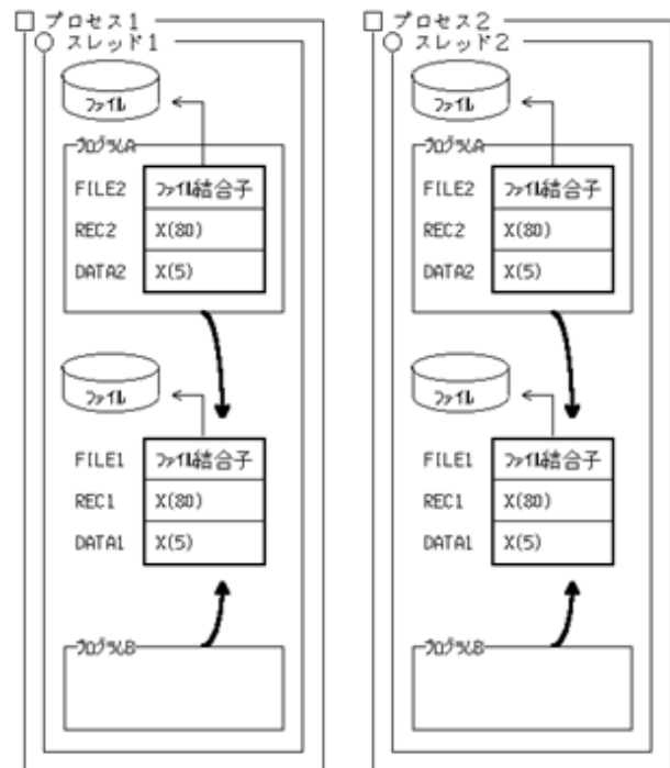
図18.2 シングルスレッドプログラム
