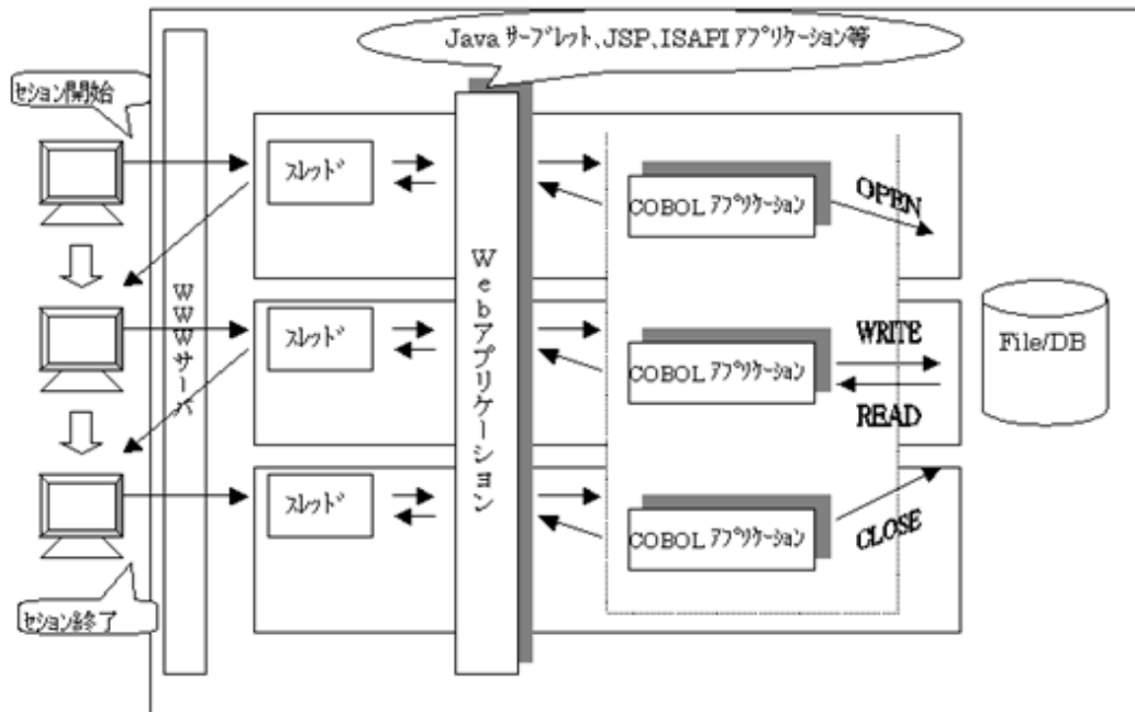
[実行単位を引き継ぐ場合]
