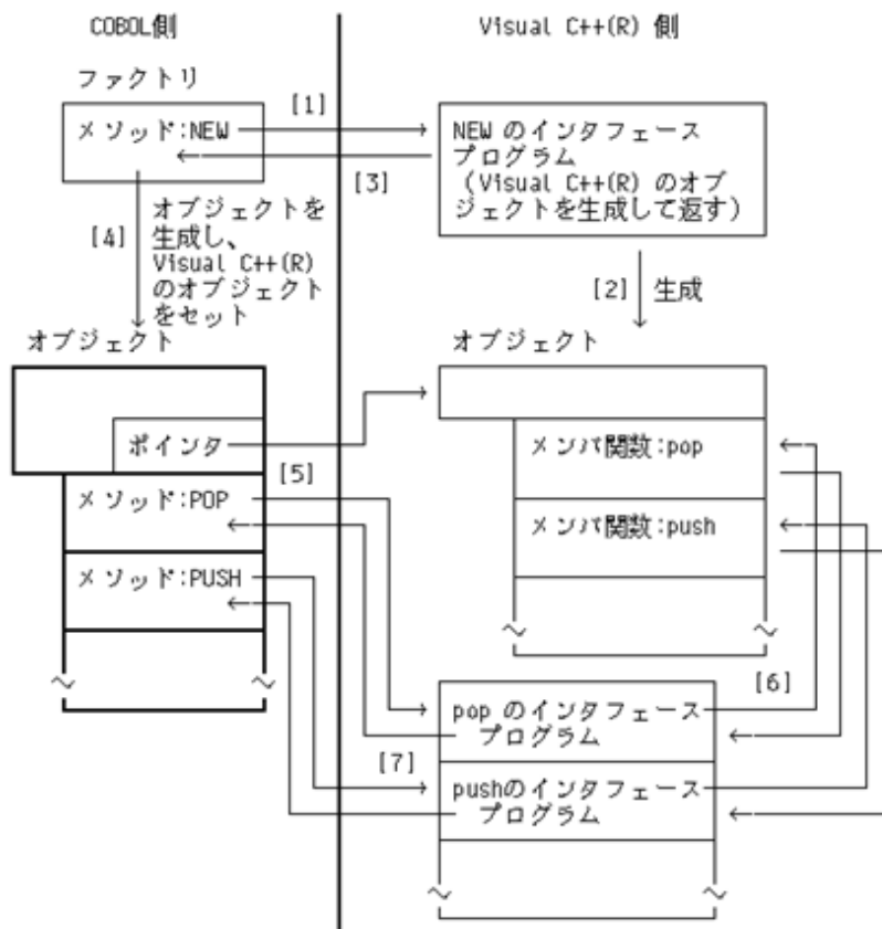
図16.13 実行時の制御の流れ
