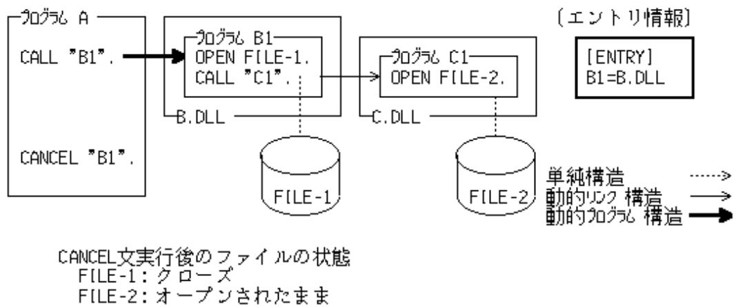
図10.7 キャンセルされる副プログラムが動的リンク構造の副プログラムを呼び出している場合
