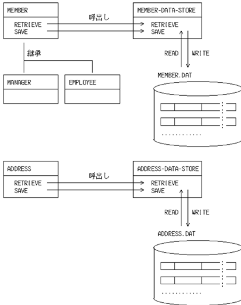
図16.20 索引ファイル操作クラスとの関係
