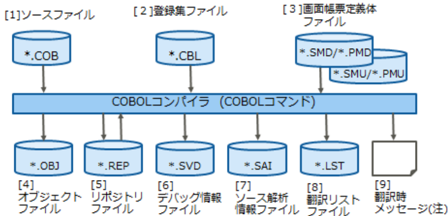
図3.1 COBOLコンパイラが使用するファイルの関係
