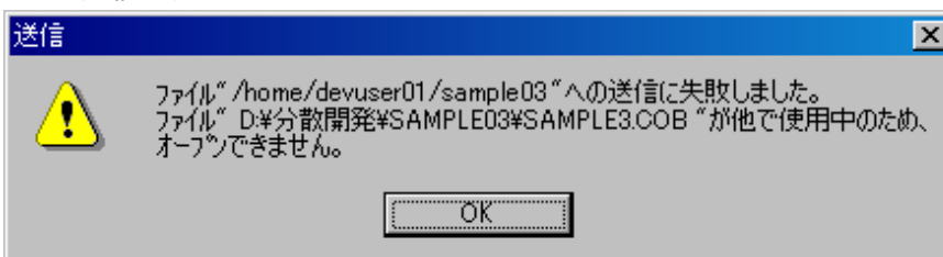
図5.2 送信エラー
