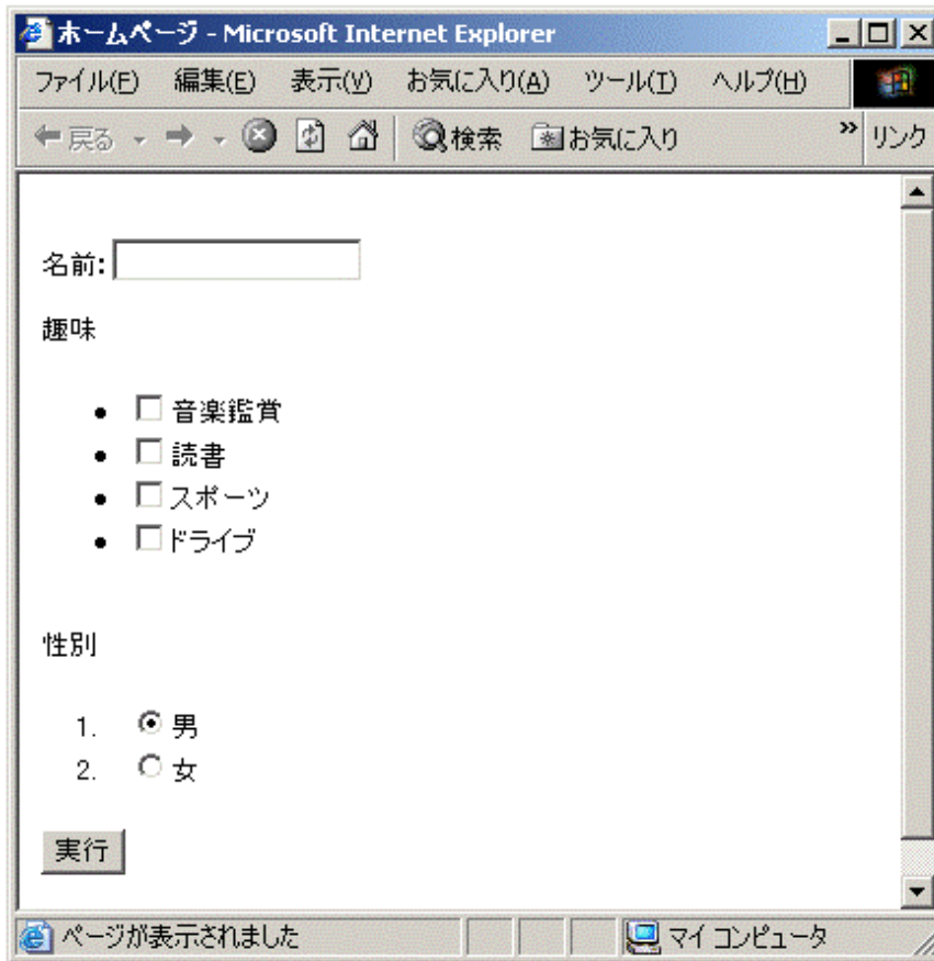
図4.19 html表示例
