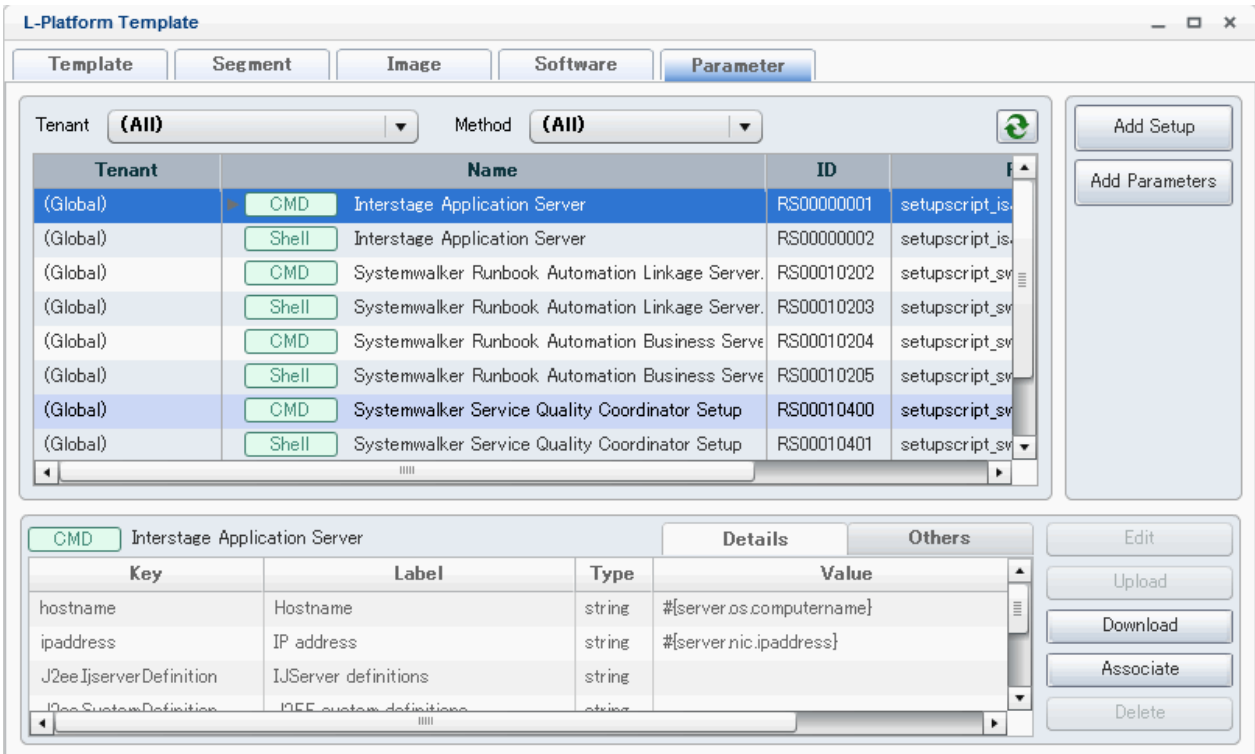
Figure 7.2 Parameter tab
