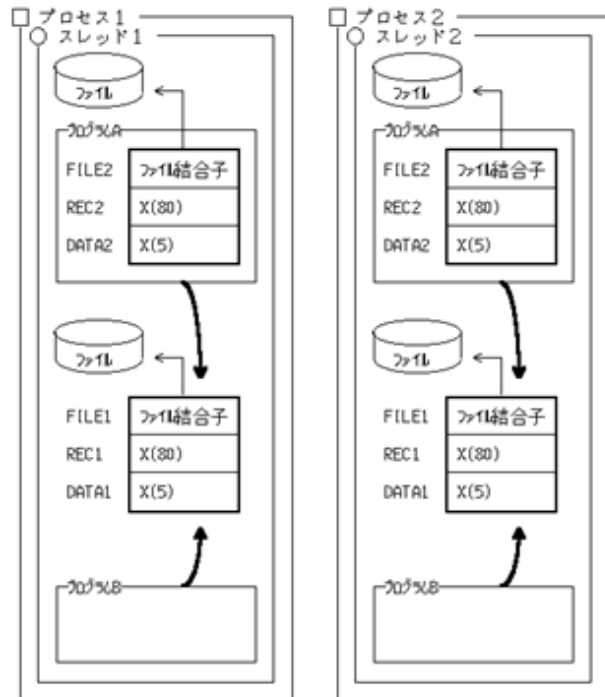
図18.2 シングルスレッドプログラム
