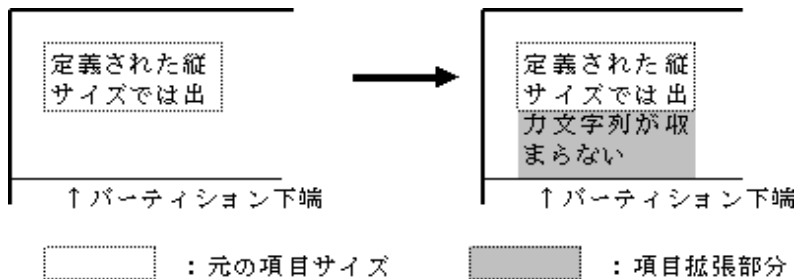
図4.23 項目の拡張
