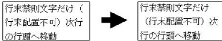
図4.17 行末禁則
