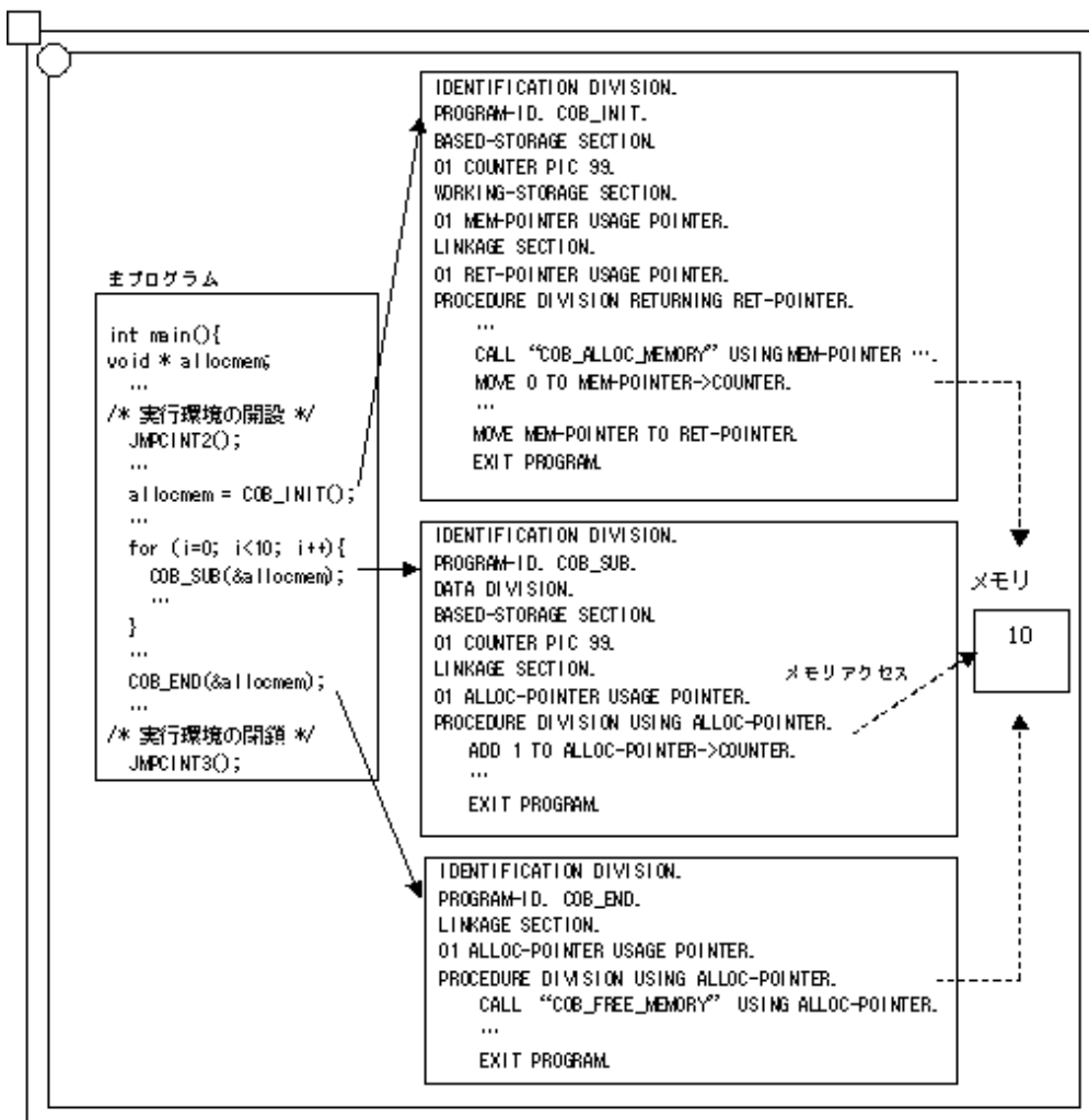
図I.2 シングルスレッドモードにおけるメモリ割当て(主プログラムが他言語)
