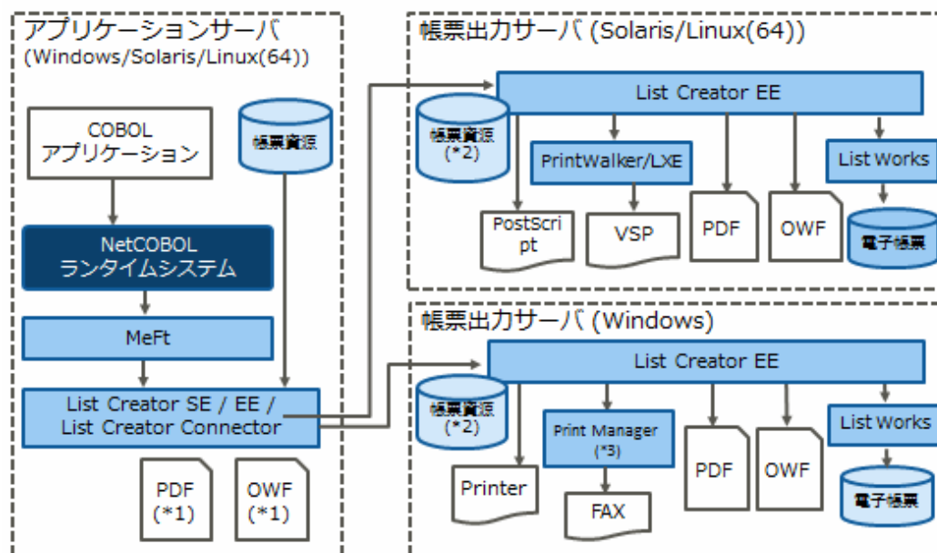
図8.3 List Creator連携(COBOLアプリケーション連携機能)
