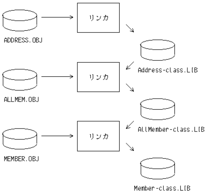
図17.10 インポートライブラリとリンク処理の順序
