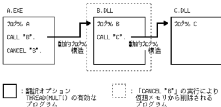
(c) プログラム B とプログラム C が動的プログラム構造
