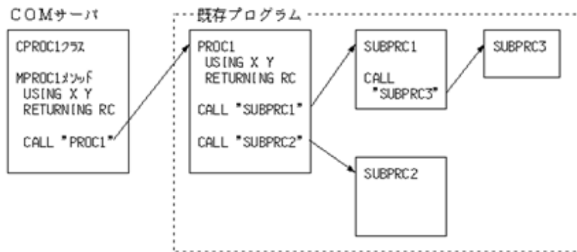
図28.9 手続き型プログラムをCOMサーバ化する例
