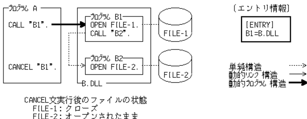
図10.11 キャンセルされる副プログラムが単純構造の副プログラムを呼び出している場合
