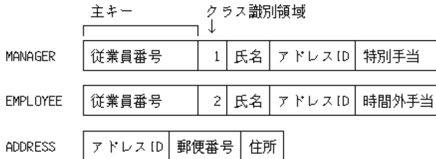
図17.19 索引ファイル中のレコード
