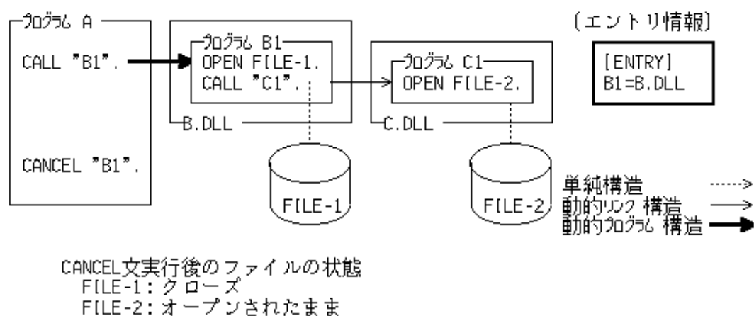
図10.12 キャンセルされる副プログラムが動的リンク構造の副プログラムを呼び出している場合
