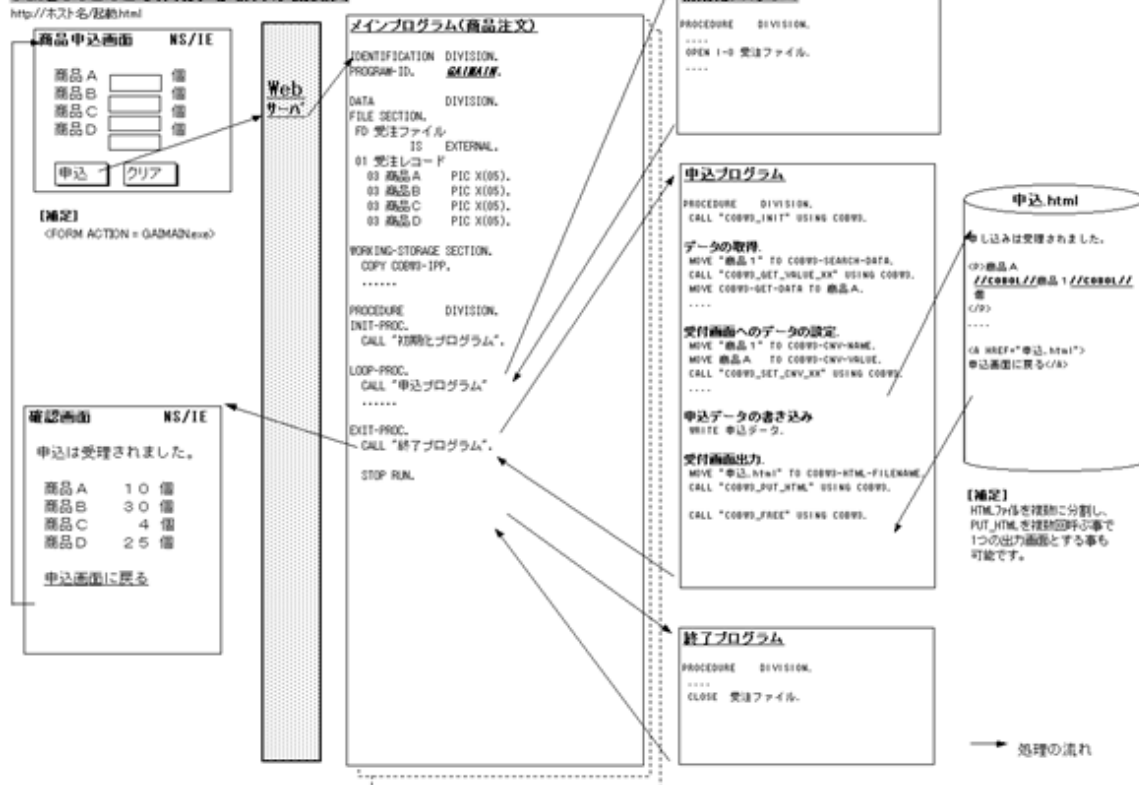
CGIをCOBOLで作成する場合の概念図
