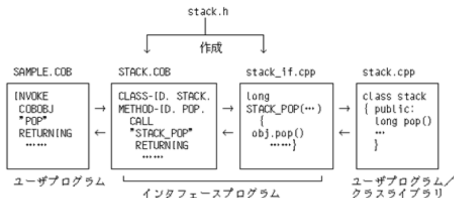
図17.11 インタフェースプログラムのイメージ
