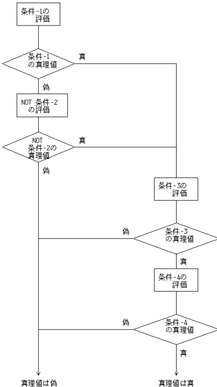
図6.4 “(条件-1 OR NOT 条件-2) AND 条件-3 AND 条件-4”の評価順序
