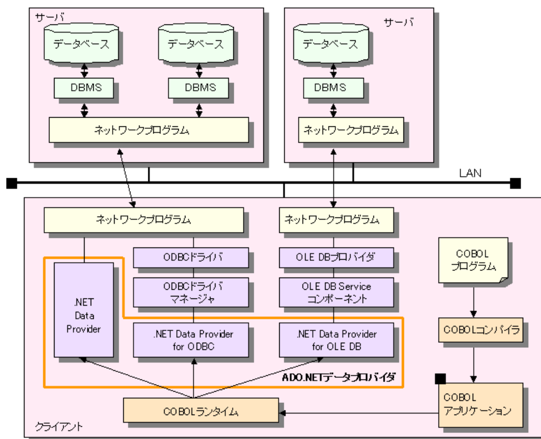
図: ADO.NET 接続でのデータベースアクセスの概要図
