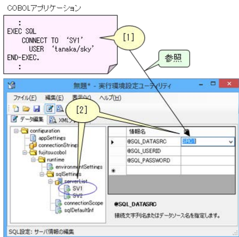
図:アプリケーション構成ファイルを使用しサーバ名を指定して実行する方法
