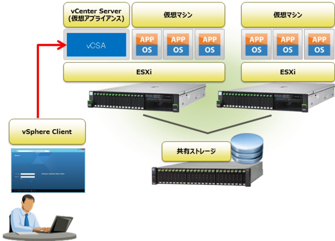
図1 vSphere 8のシステム構成イメージ
