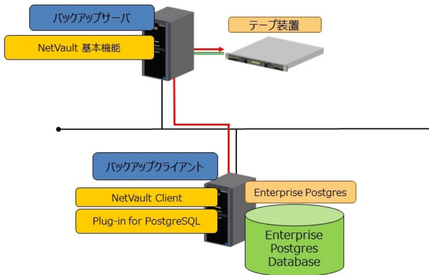
Enterprise Postgres をバックアップクライアントとしてバックアップサーバに接続されたテープ装置へオンラインバックアップ
